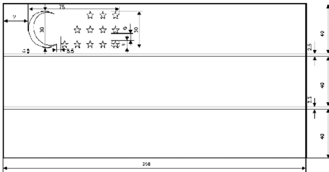
Sxematik rasmi
